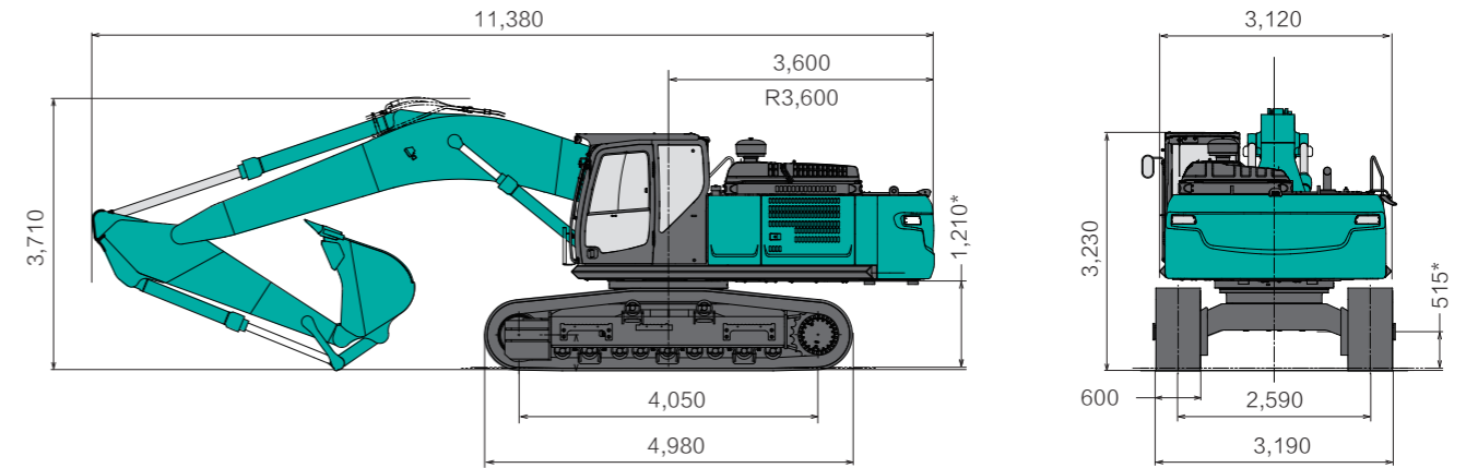
标准2.6m小臂。*记号表示不包括履带板突出部分。
