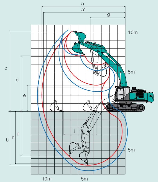
标准2.6m小臂。*记号表示不包括履带板突出部分。
